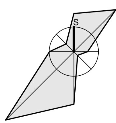
Větrná růžice:
