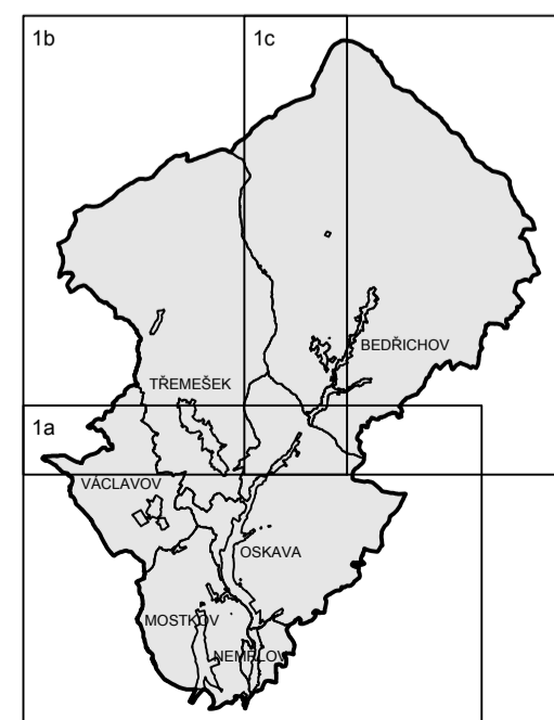
Klad sekcí:
